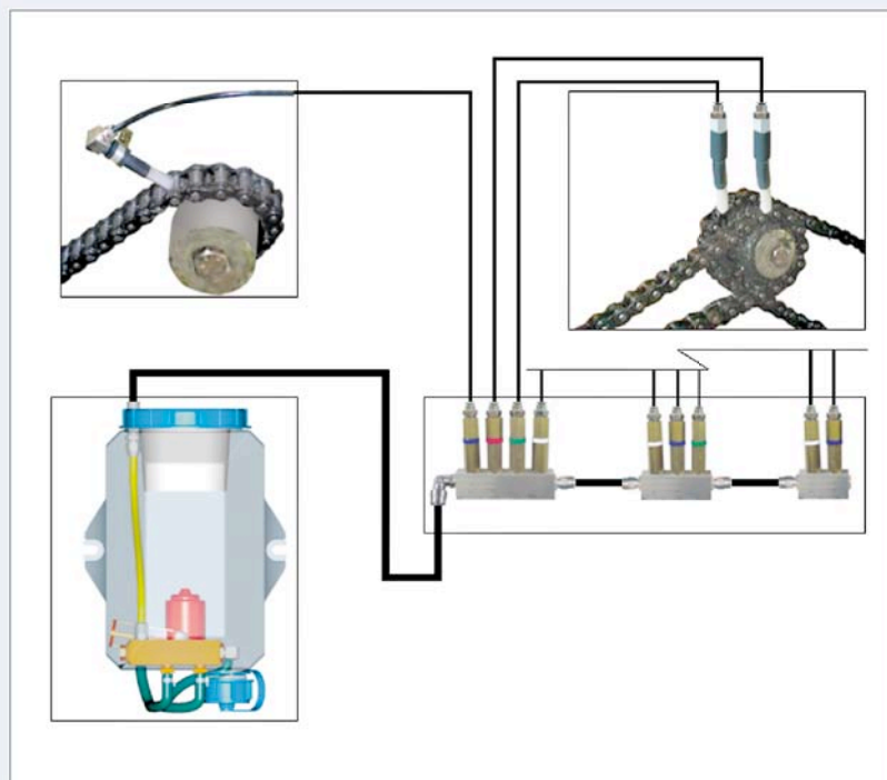
EOS—система смазки
